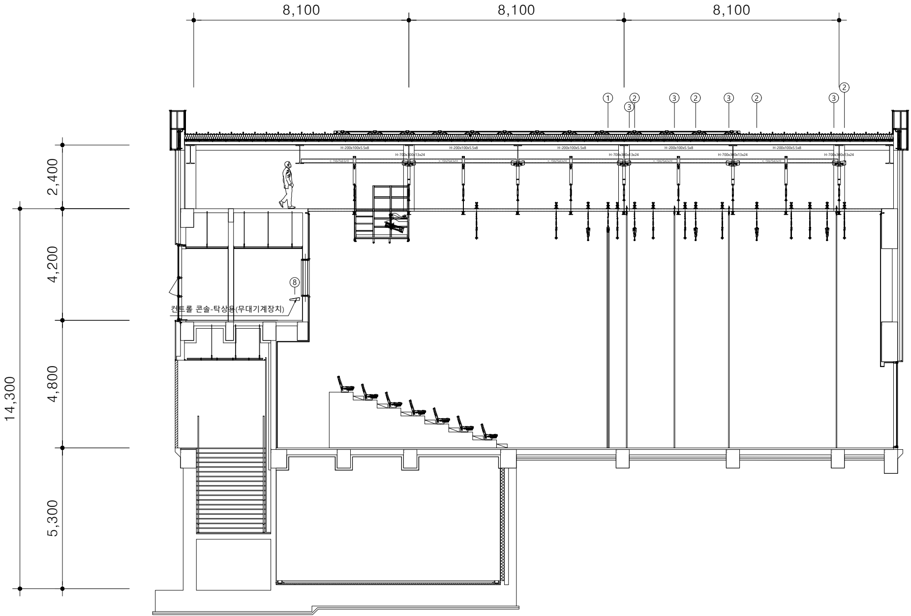
블랙박스 무대장치 단면도
